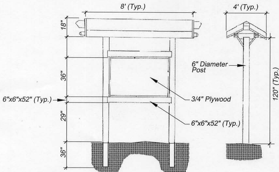
TYPICAL KIOSK
